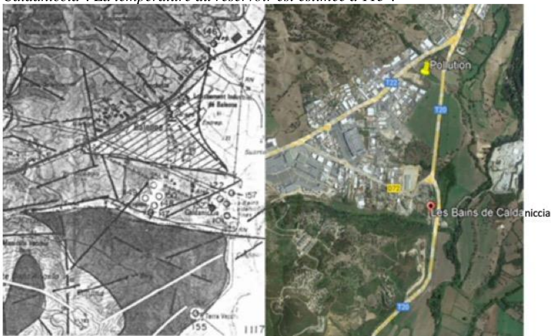
Rapprochement aquifère et terrain pollué : à gauche les zones de fracture d'une arène granodioritique qui renferme une eau sulfurée sodique chaude qui alimente les "bains de Caldaniccia". La température du réservoir est estimée à 115°.
